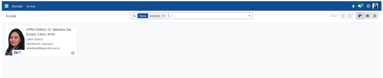
Gambar 8. Profil kontak
