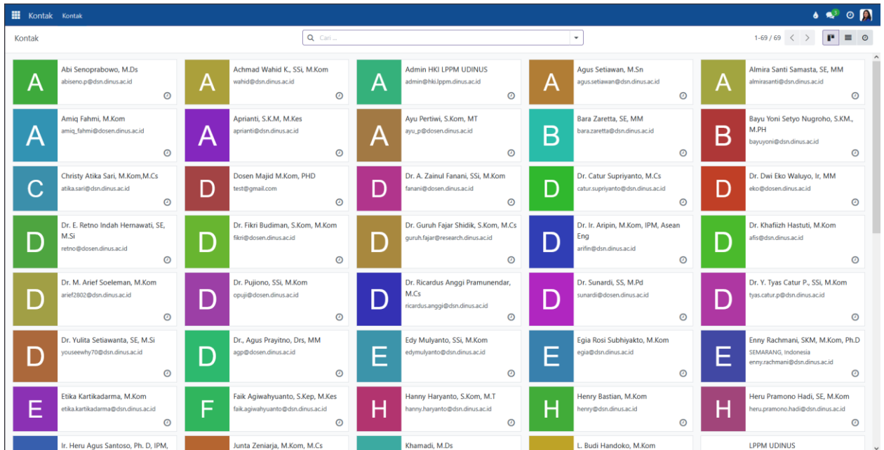
Gambar 6. Menu kontak
